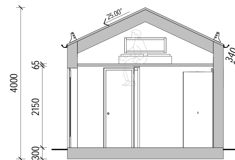
SEKTION A-A
